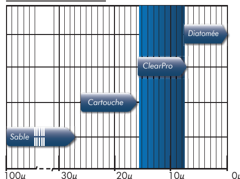
Niveau de filtration
