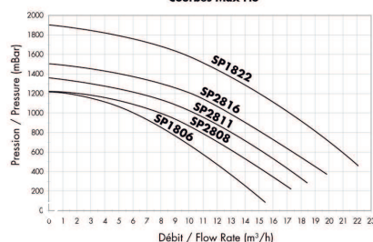
Courbes Max Flo®
