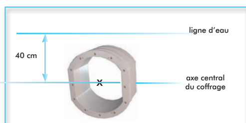
Insert laiton côté intérieur du bassin
